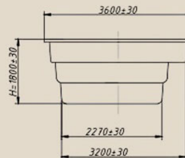
Вид Б
