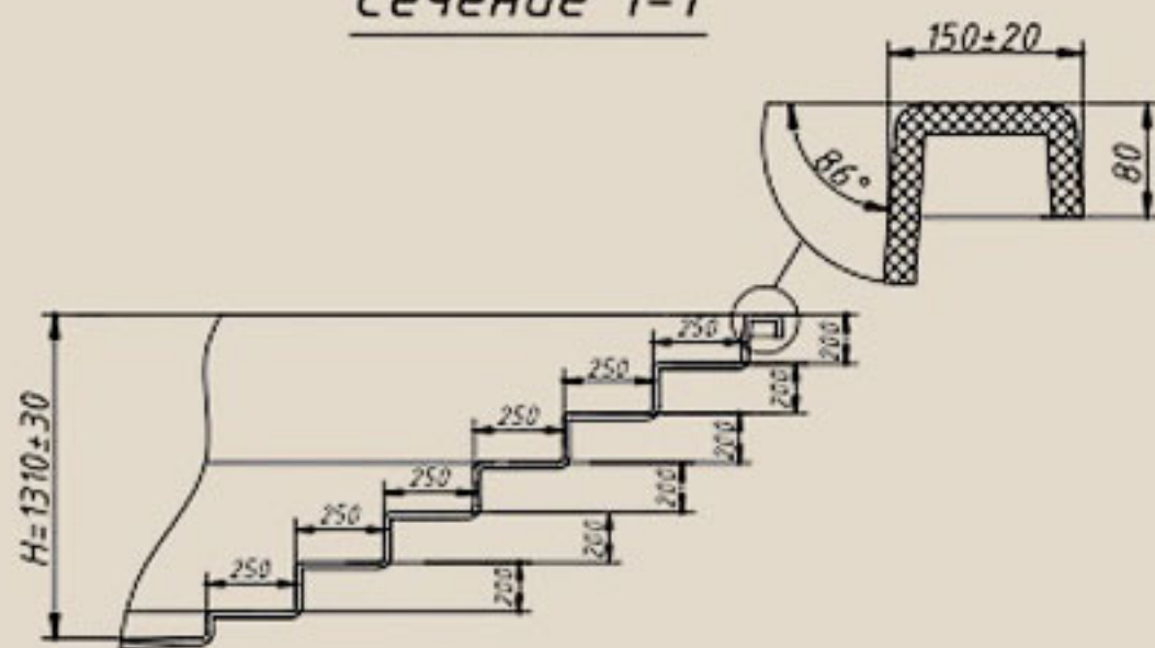
Сечение 1-1
