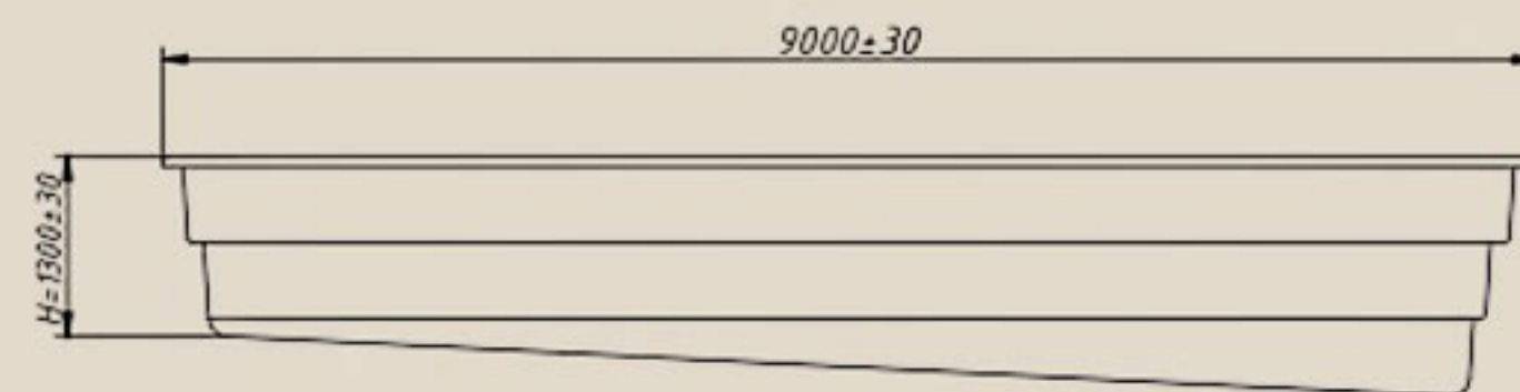
Вид Г
