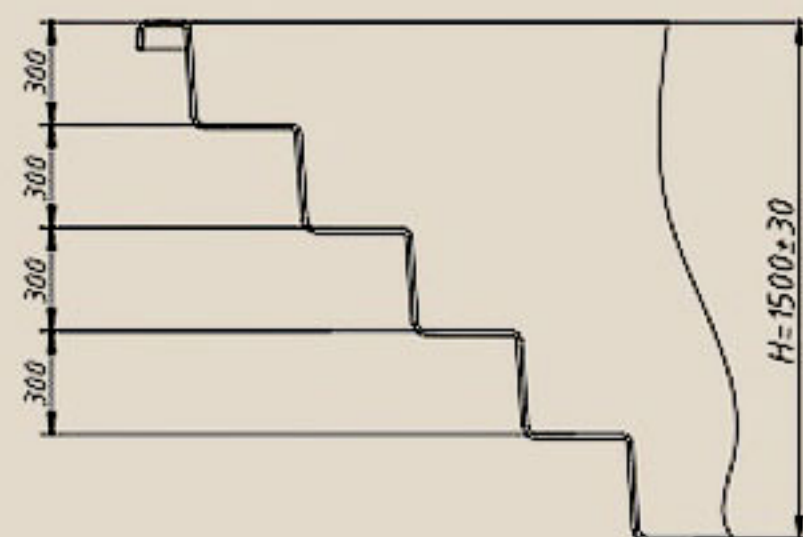
Сечение 1-1
