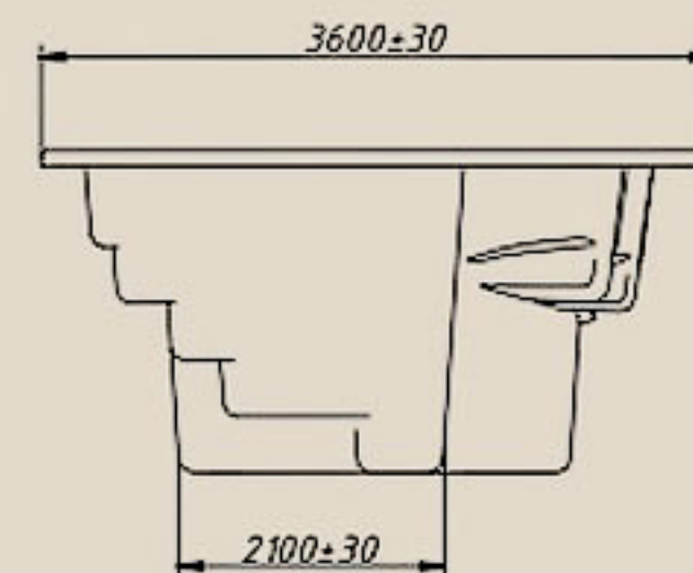
Вид В
