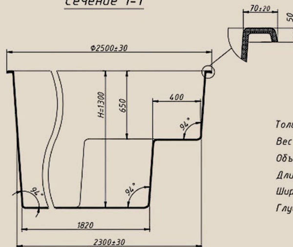
Сечение 1-1
