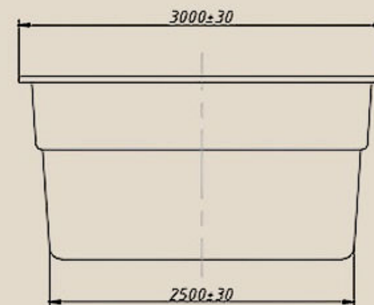
Вид Б
