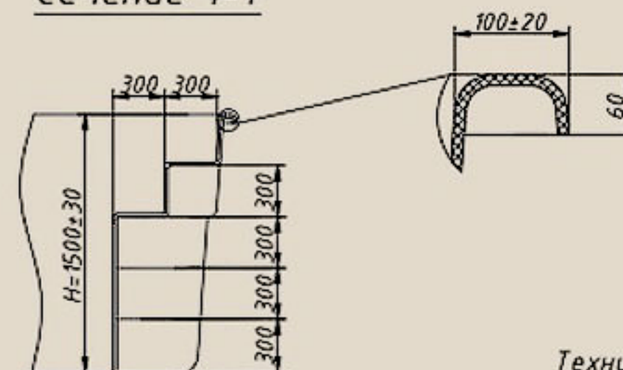
Сечение 1-1
