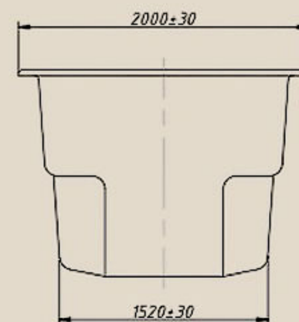
Вид Б
