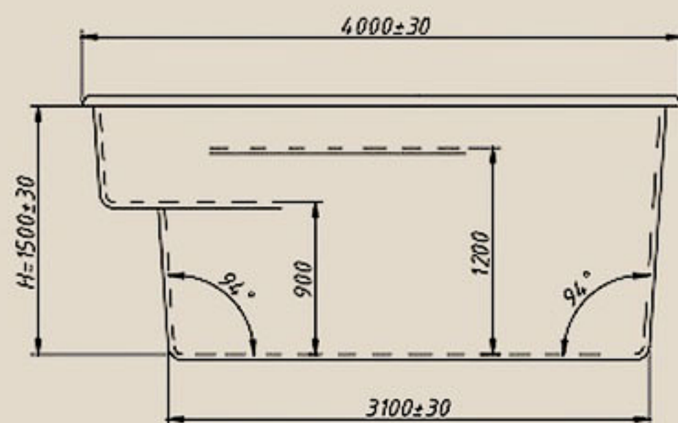
Вид А
