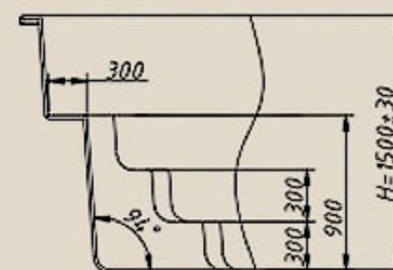
Сечение 1-1
