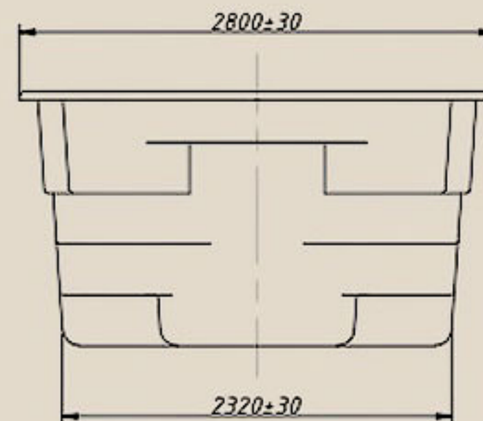
Вид Б
