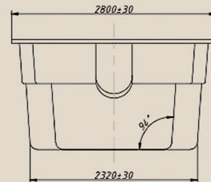
Вид В
