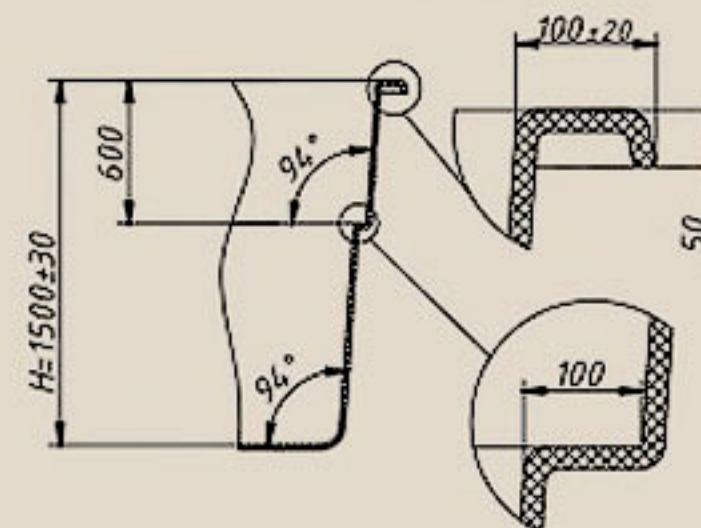
Сечение 2-2
