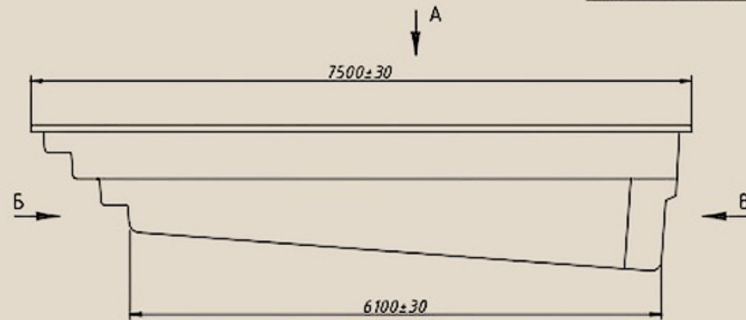
Вид А
