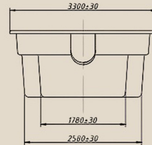
Вид Б
