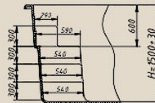
Сечение 2-2
